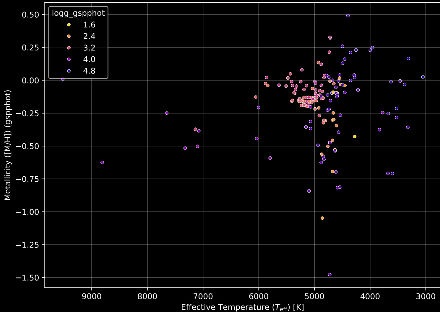
APOGEE DR17 Field: [190-19] Stellar Population Parameters (n= 179)
